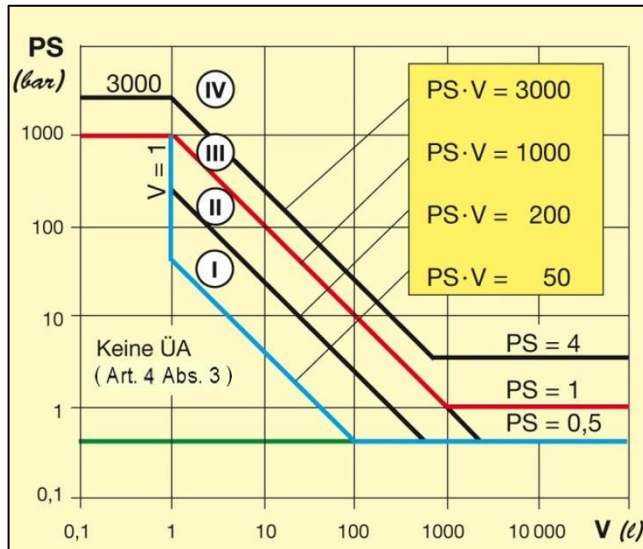
Bild 7: Diagramm 2 nach Anhang II der DGRL für Behälter für Gase (auch überhitzte Flüssigkeiten) der Fluidgruppe 2 mit Prüfstufen für die für die wiederkehrende Prüfung (§16 BetrSichV)
